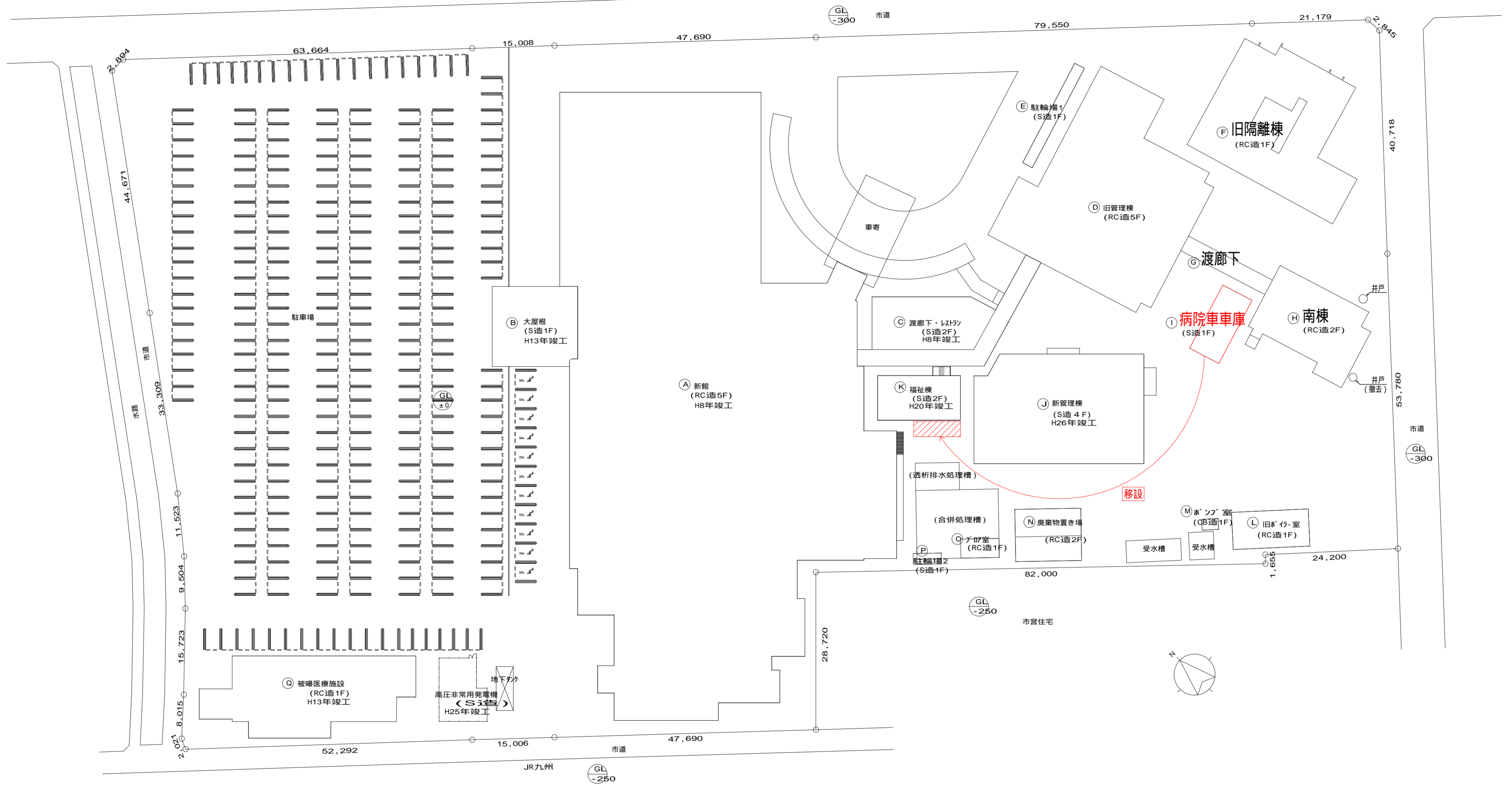
配置図 1:500
